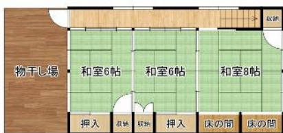
2階平面図
