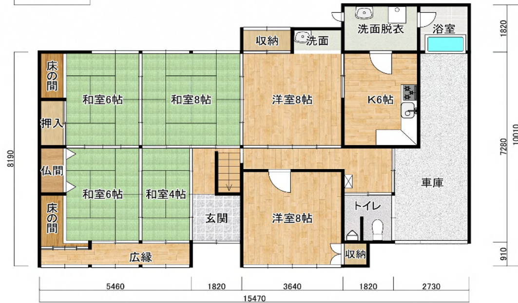
1階平面図
